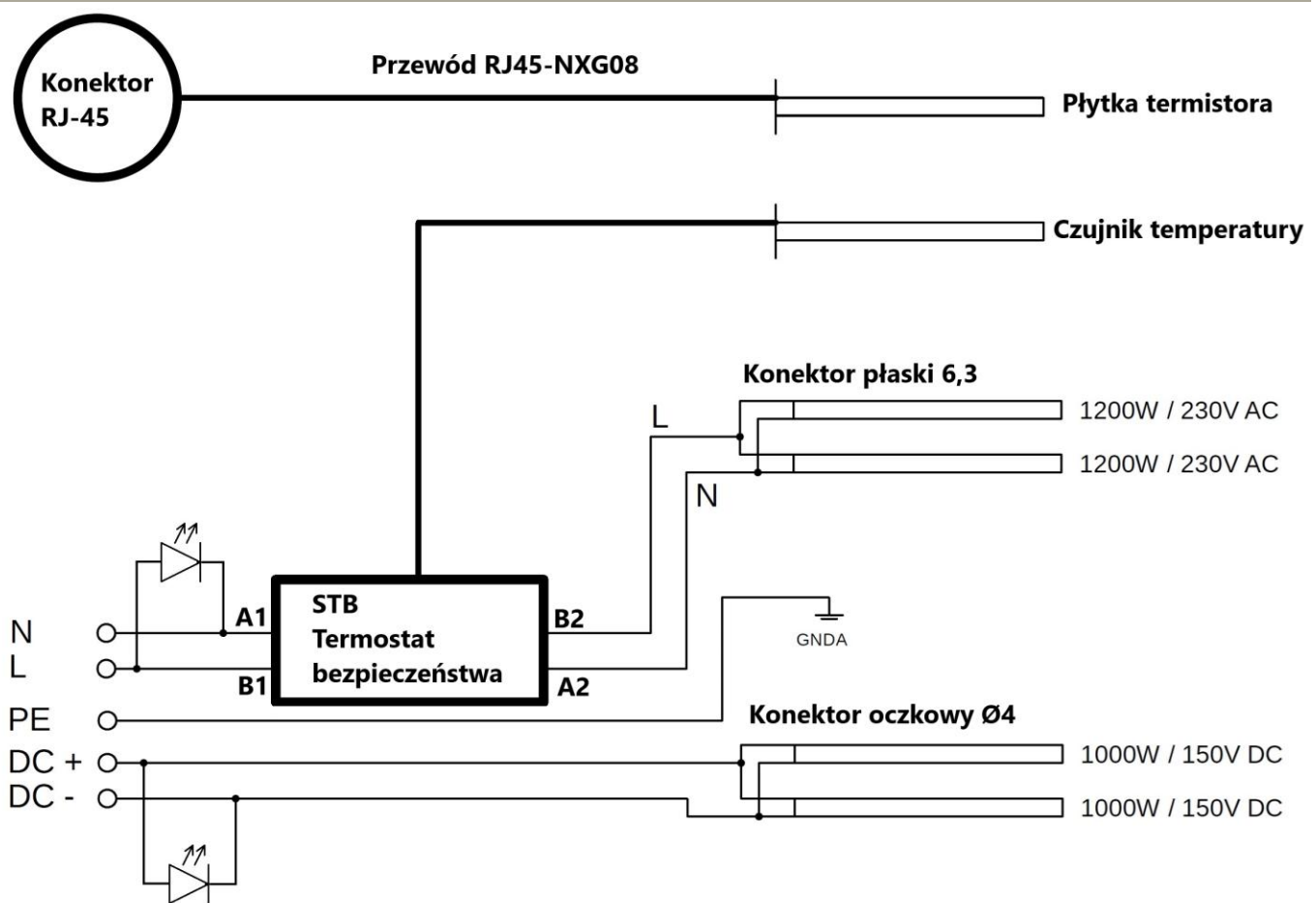
Rys. 6. Schemat instalacji elektrycznej ogrzewacza solarnego NORDIC PV.
