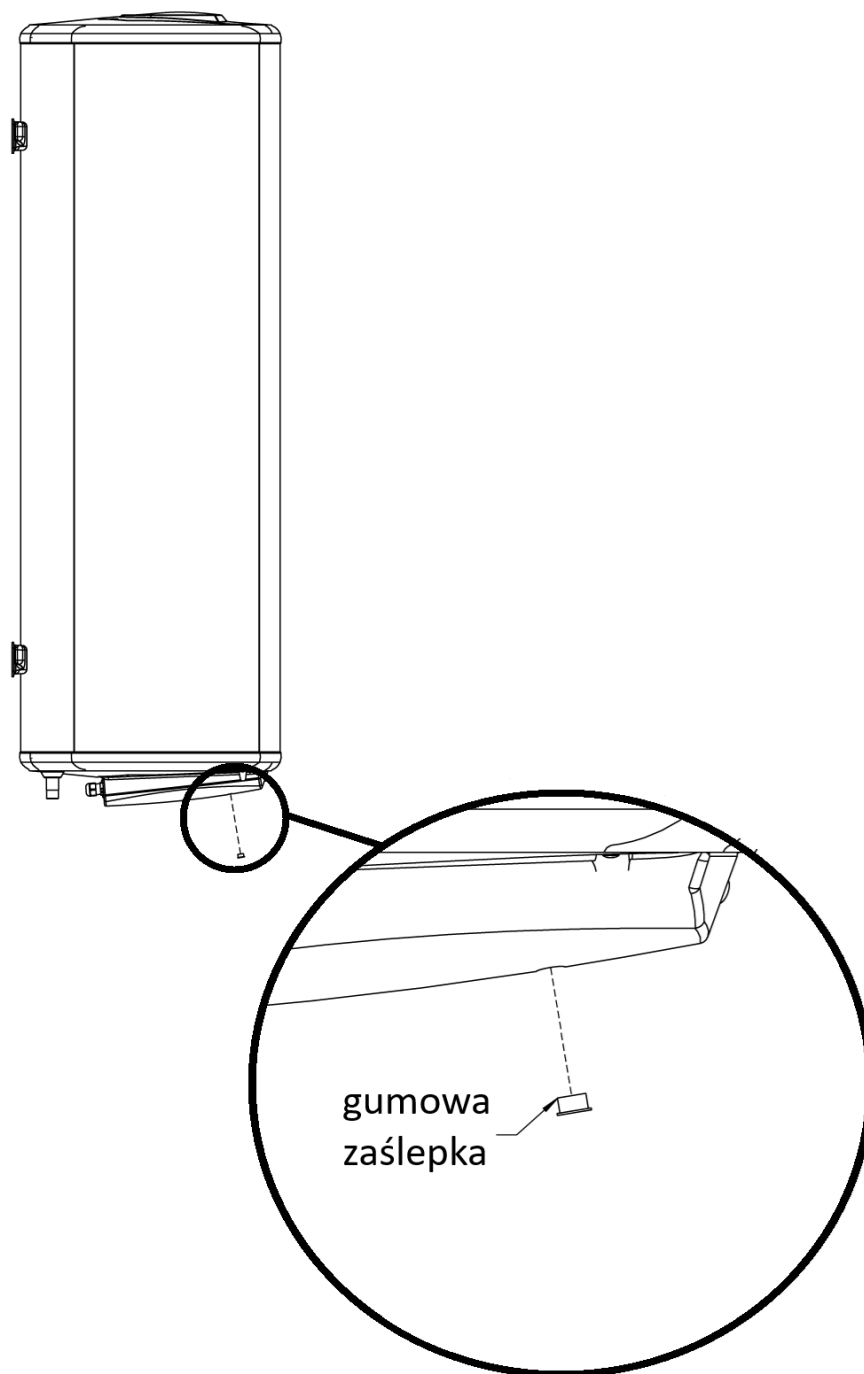
Rys. 2. Demontaż gumowej zaślepki ogranicznika temperatury STB.
